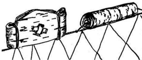
Figur 1. Näverflöten använda vid flundrefiske, Rågö, Estland. Efter Söderbäck 1940.
