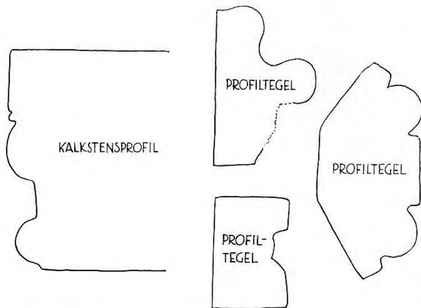
Fig. 5. Skärningar av en kalkstenslist och profiltegel.
