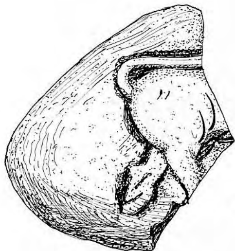
Fig. 2 a. Tegning af Skiferstenen fra Sigtuna. Ca dobbelt størrelse.
