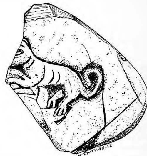
Fig. 2 b. Tegning af Skiferstenen, den anden side. Ca dobbelt størrelse.
