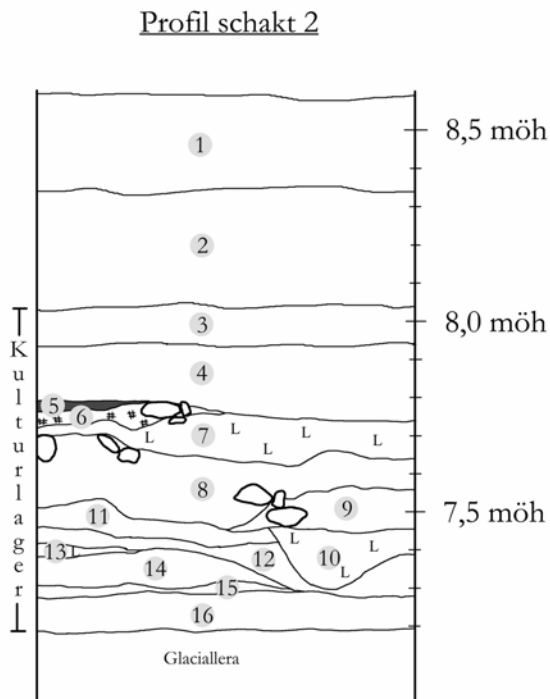
Figur 2 Profilritning i skala 1:40
