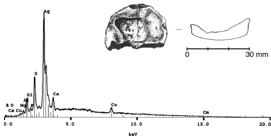
Fig. 5. Skärvel, Birkas stadsvall, och diagram från XRF-analys av metalldroppe vid ytan visande den kraftiga silvertoppen samt ett lätt kopparutslag till höger. Notera ovasidans fördjupning. Teckning och analys författaren.
