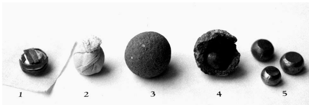
Fig. 2. Rekonstruerad arbetsgång vid lödning av vikter i smältkolor: en järnkärna smids till önskad form. Kärna och lod (1) knyts in i ett sammanhållande stycke linne (2) varefter knytet packas in i magrad lera (3). Den torra lerkulan läggs i härden och hettas upp. Lodet smälter och rinner ut runt kärnan. Därefter tas kulan ur härden och slås sönder efter avsvälning (4). Den färdiga vikten kan tas ut (5). Foto författaren.
