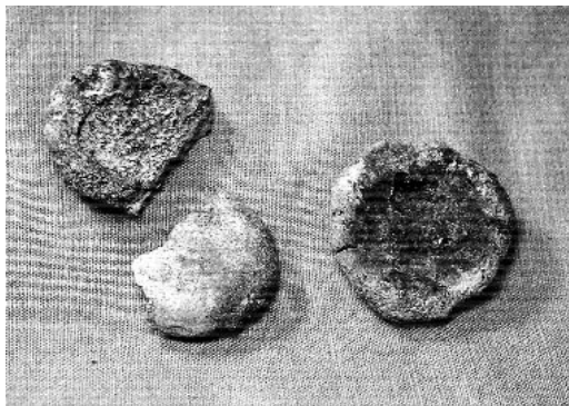
Fig. 3. Skärvlar, Sigtuna. Fragmentet till vänster har en stor nedflussad porig fördjupning i ytan, omfattande större delen av ovansidan. Plattan till höger har en betydligt mindre depression. Foto författaren.
